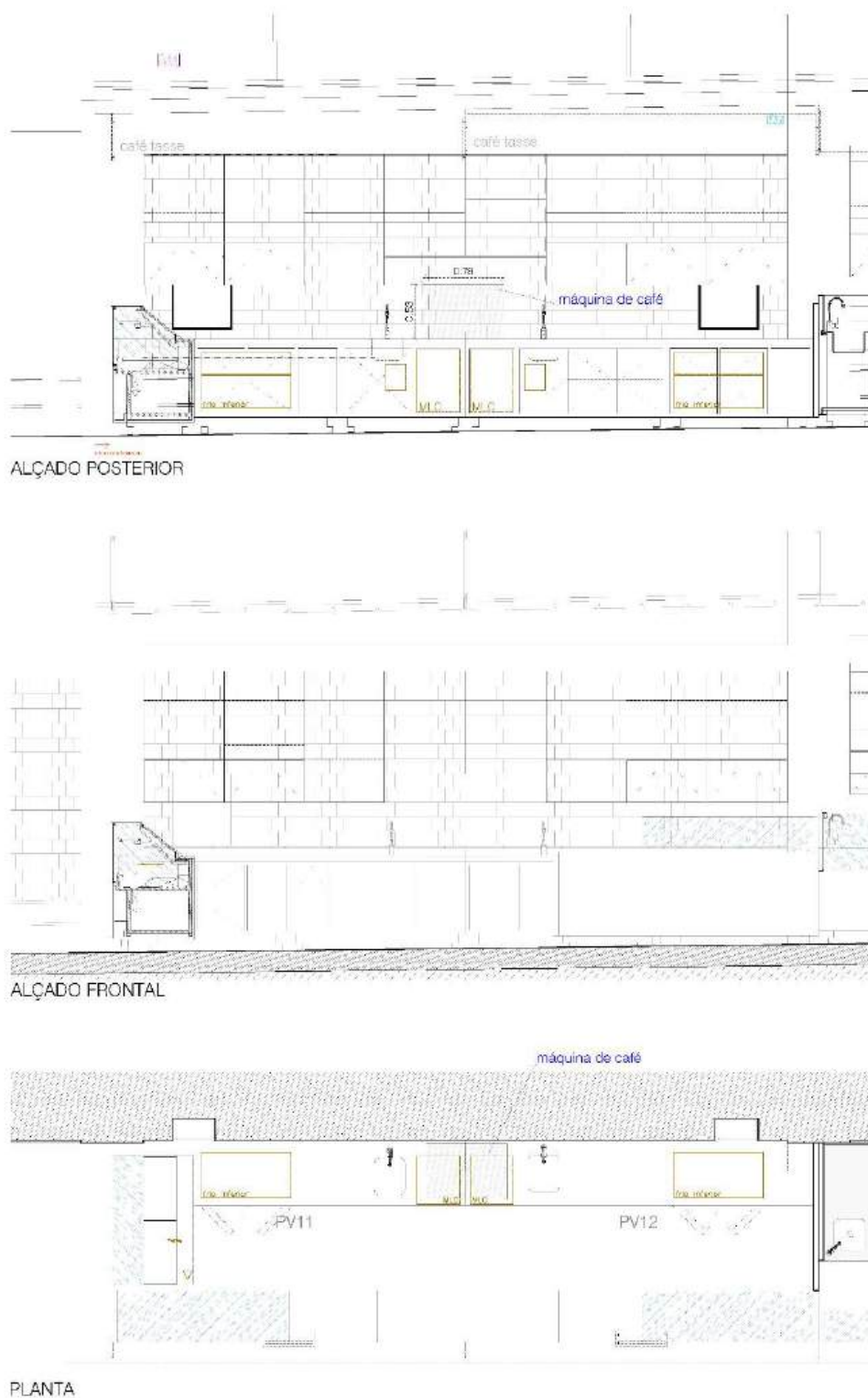
Desenho 1.01 – Adaptação móvel expositor (Máquina de Café)
