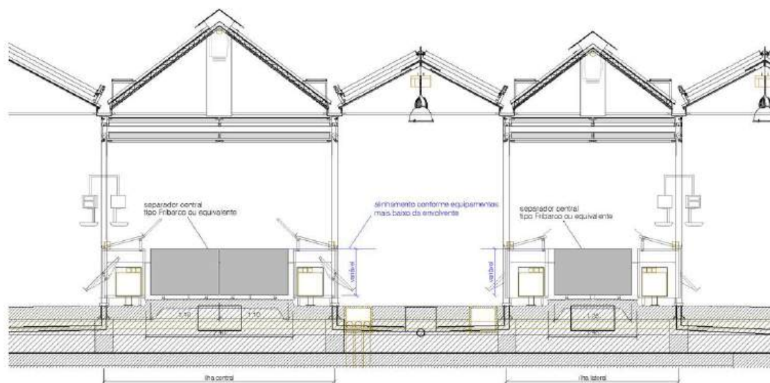
CORTE 1
